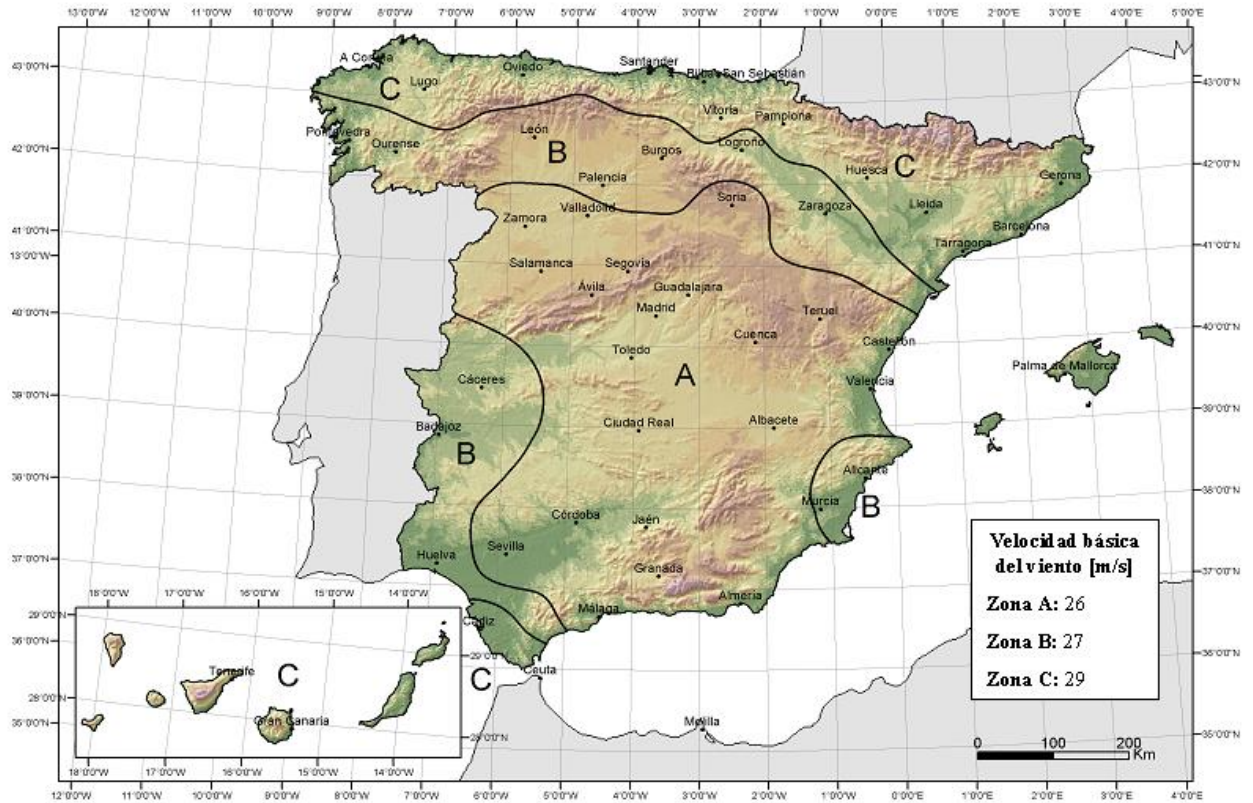
Figura 2.5 Zonas eólicas
